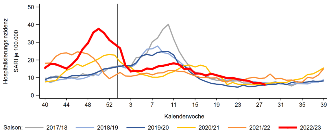
Abb. 5: Wöchentlich Inzidenz je 100.000 Einwohner der neu im Krankenhaus aufgenommenen SARI-Fälle (ICD-10-Codes J09-J22), in den Saisons 2017/18 bis 2022/23 (bis zur 28. KW 2023), Daten aus 70 Sentinelkliniken. Der senkrechte Strich markiert jeweils die 1. KW des Jahres.
