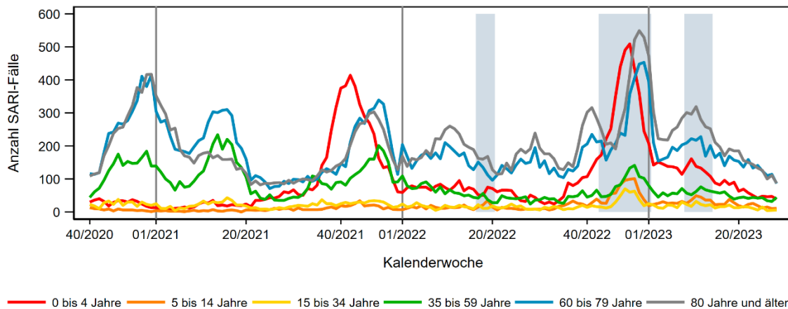
Abb. 6: Wöchentliche Anzahl der neu im Krankenhaus aufgenommenen SARI-Fälle (ICD-10-Codes J09 – J22) nach Altersgruppen, von der 40. KW 2020 bis zur 28. KW 2023, Daten aus 70 Sentinellkliniken. Der senkrechte Strich markiert jeweils die 1. KW des Jahres, der Zeitraum der Grippewelle ist grau hinterlegt.
