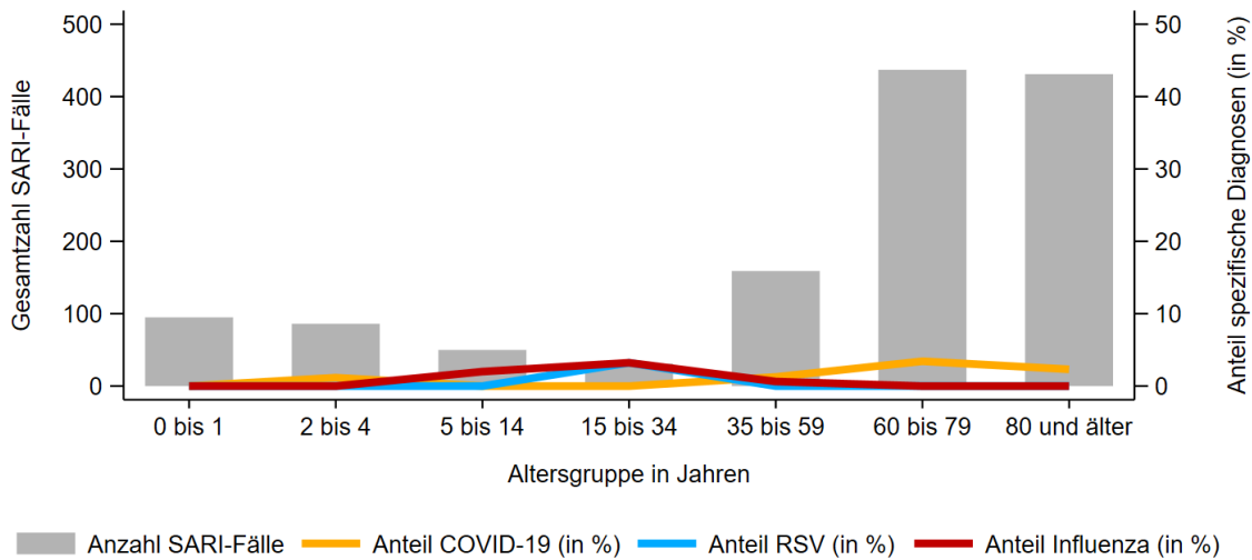
Abb. 8: Anzahl der von der 25. KW bis zur 28. KW 2023 neu im Krankenhaus aufgenommenen SARI-Fälle (ICD-10-Codes J09 – J22) nach Altersgruppe sowie Anteil der Fälle mit einer zusätzlichen COVID-19-Diagnose (ICD-10-Code U07.1!), einer RSV-Diagnose (ICD-10 Codes J12.1, J20.5, J21.0) bzw. einer Influenza-Diagnose (ICD-10-Code J10) unter SARI-Fällen.
