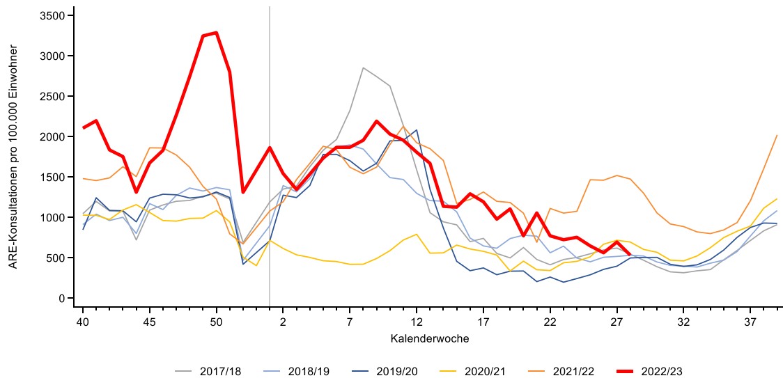
Abb. 2: Werte der Konsultationsinzidenz gesamt in Deutschland pro 100.000 Einwohner in den Saisons 2017/18 bis 2022/23 (bis zur 28. KW 2023). Der senkrechte Strich markiert die 1. KW des Jahres.
