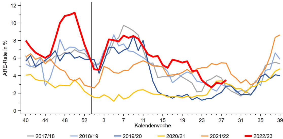
Abb. 1: Vergleich der für die Bevölkerung in Deutschland geschätzten ARE-Raten (in Prozent) in den Saisons 2017/18 bis 2022/23 (bis zur 28. KW 2023). Der senkrechte Strich markiert den Jahreswechsel.
