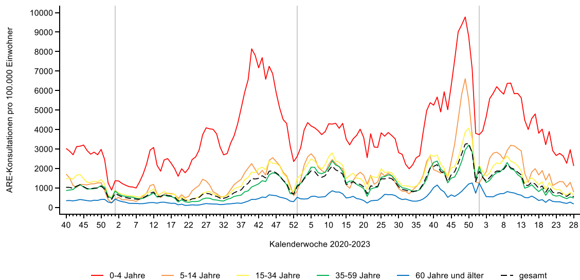
Abb. 3: Werte der Konsultationsinzidenz von der 40. KW 2020 bis zur 28. KW 2023 in fünf Altersgruppen und gesamt in Deutschland pro 100.000 Einwohner in der jeweiligen Altersgruppe. Der senkrechte Strich markiert jeweils die 1. KW des Jahres.
