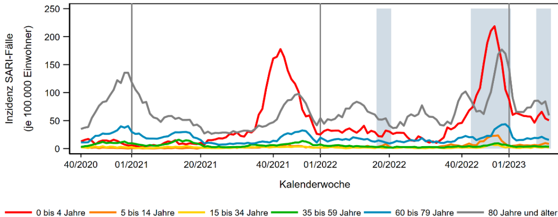
Abb. 9: Wöchentliche Inzidenz je 100.000 Einwohner der neu im Krankenhaus aufgenommenen SARI-Fälle (ICD-10-Codes J09 – J22) nach Altersgruppen, von der 40. KW 2020 bis zur 12. KW 2023, Daten aus 71 Sentinelkliniken. Der senkrechte Strich markiert jeweils die 1. KW des Jahres, der Zeitraum der Grippewelle ist grau hinterlegt.
