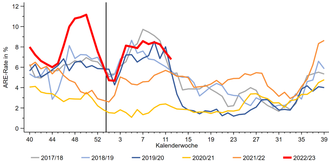
Abb. 1: Vergleich der für die Bevölkerung in Deutschland geschätzten ARE-Raten (in Prozent) in den Saisons 2017/18 bis 2022/23 (bis zur 12. KW 2023). Der senkrechte Strich markiert den Jahreswechsel.
