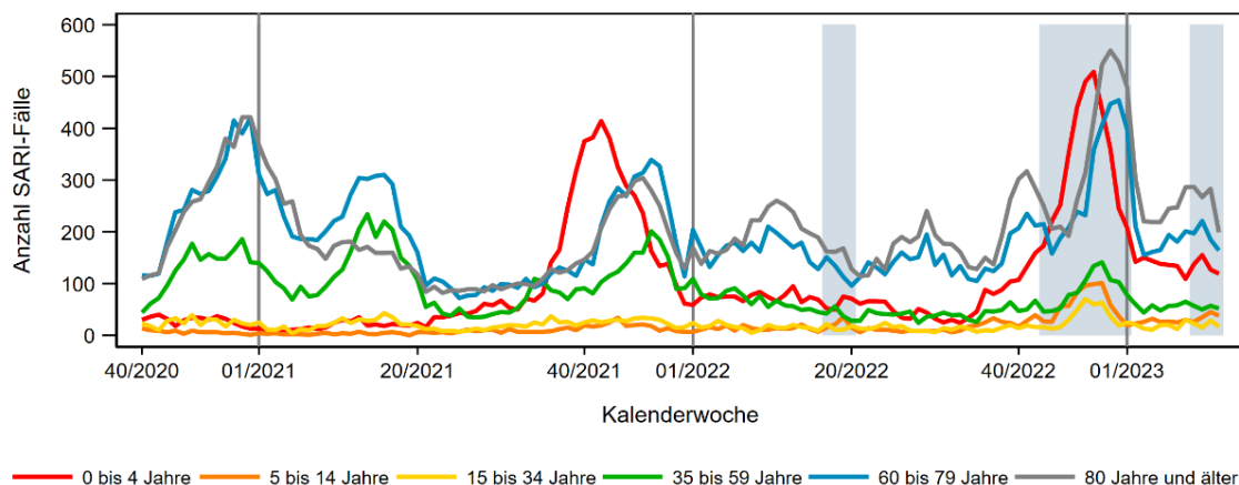
Abb. 8: Wöchentliche Anzahl der neu im Krankenhaus aufgenommenen SARI-Fälle (ICD-10-Codes J09 – J22) nach Altersgruppen, von der 40. KW 2020 bis zur 12. KW 2023, Daten aus 71 Sentinelkliniken. Der senkrechte Strich markiert jeweils die 1. KW des Jahres, der Zeitraum der Grippewelle ist grau hinterlegt.
