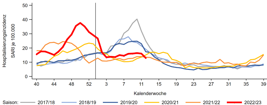
Abb. 7 Wöchentlich Inzidenz je 100.000 Einwohner der neu im Krankenhaus aufgenommenen SARI-Fälle (ICD-10-Codes J09-J22), in den Saisons 2017/18 bis 2022/23 (bis zur 12. KW 2023), Daten aus 71 Sentinelkliniken. Der senkrechte Strich markiert jeweils die 1. KW des Jahres.
