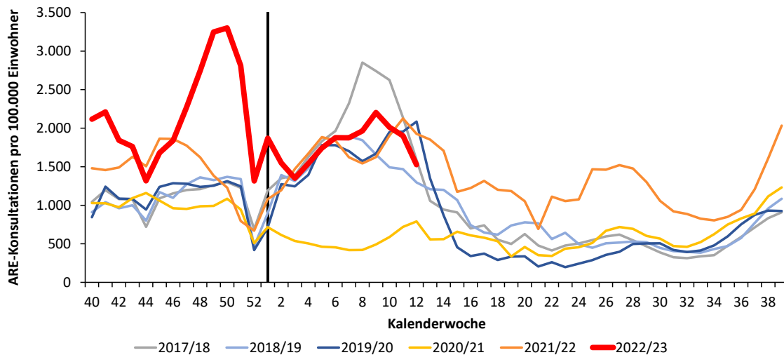
Abb. 2: Werte der Konsultationsinzidenz gesamt in Deutschland pro 100.000 Einwohner in den Saisons 2017/18 bis 2022/23 (bis zur 12. KW 2023). Der senkrechte Strich markiert die 1. KW des Jahres.
