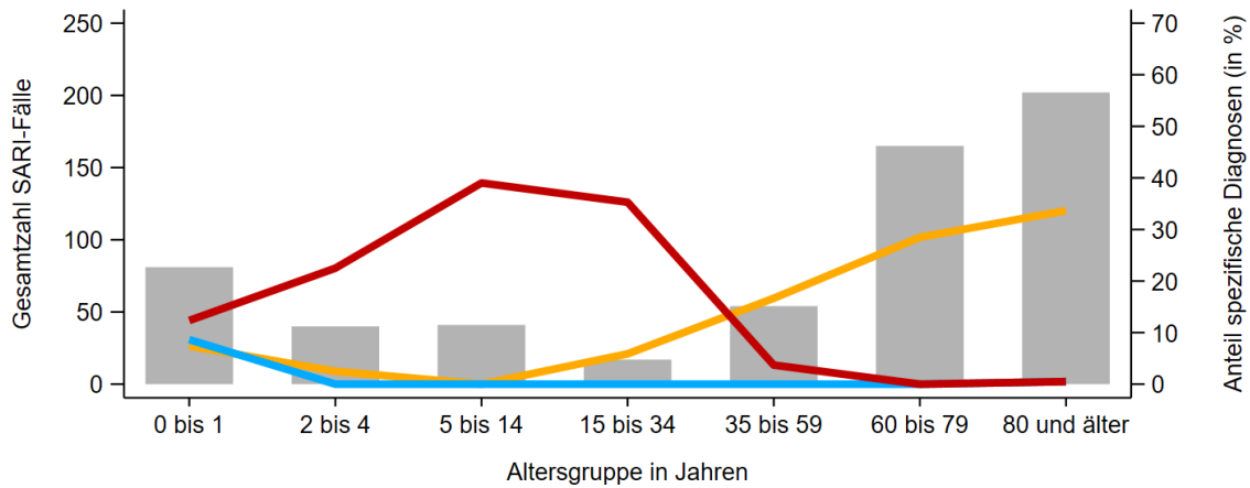
Abb. 11: Anzahl der in der 12. KW 2023 neu im Krankenhaus aufgenommenen SARI-Fälle (ICD-10-Codes J09 – J22) nach Altersgruppe sowie Anteil der Fälle mit einer zusätzlichen COVID-19-Diagnose (ICD-10-Code U07.1!), einer RSV-Diagnose (ICD-10 Codes J12.1, J20.5, J21.0) bzw. einer Influenza-Diagnose (ICD-10-Code J10) unter SARI-Fällen.
