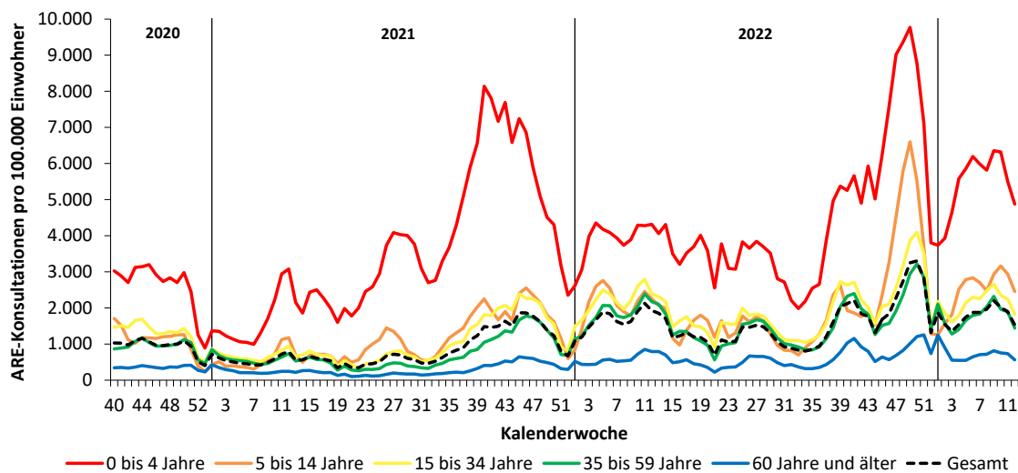
Abb. 3: Werte der Konsultationsinzidenz von der 40. KW 2020 bis zur 12. KW 2023 in fünf Altersgruppen und gesamt in Deutschland pro 100.000 Einwohner in der jeweiligen Altersgruppe. Der senkrechte Strich markiert jeweils die 1. KW des Jahres.
