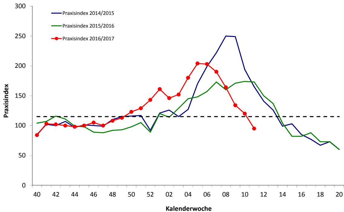
Abb. 1: Praxisindex bis zur 11. KW 2017 im Vergleich zu den Saisons 2014/15 und 2015/16 (Hintergrund-Aktivität bis zu einem Praxisindexwert von 115, gestrichelte Linie).
