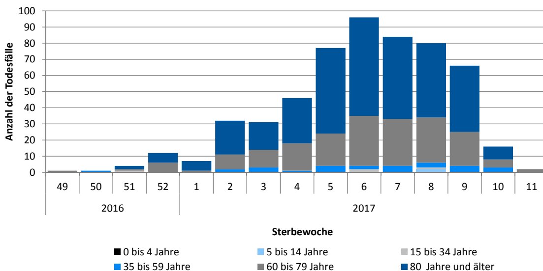
Abb. 6: Anzahl der seit der 40. KW 2016 nach IfSG an das RKI übermittelten Todesfälle mit Influenzainfektion pro Altersgruppe nach Woche, in der die Fälle verstorben sind (n = 555 Fälle mit Angabe des Sterbedatums).
